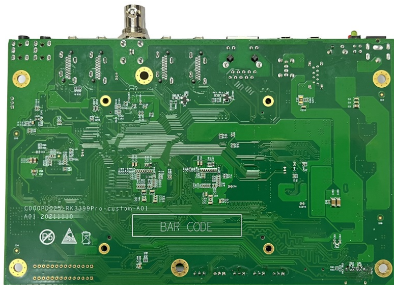
RK3399PRO 定制开发板-背面图
