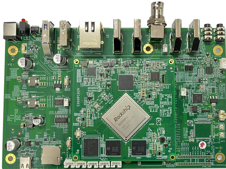
RK3399PRO 定制开发板-正面图
