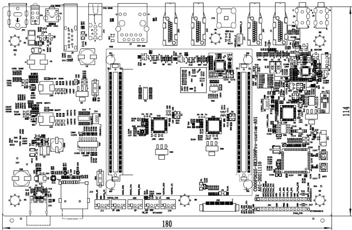
HT-RK3399Pro 定制开发板-机械尺寸图
