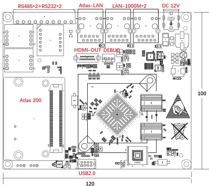
HT-RK3568 定制开发板-机械尺寸图
