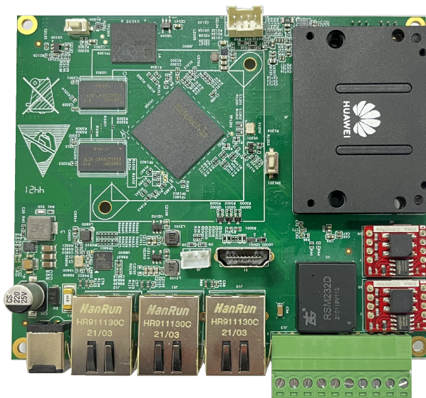
RK3568 定制开发板-正面图
