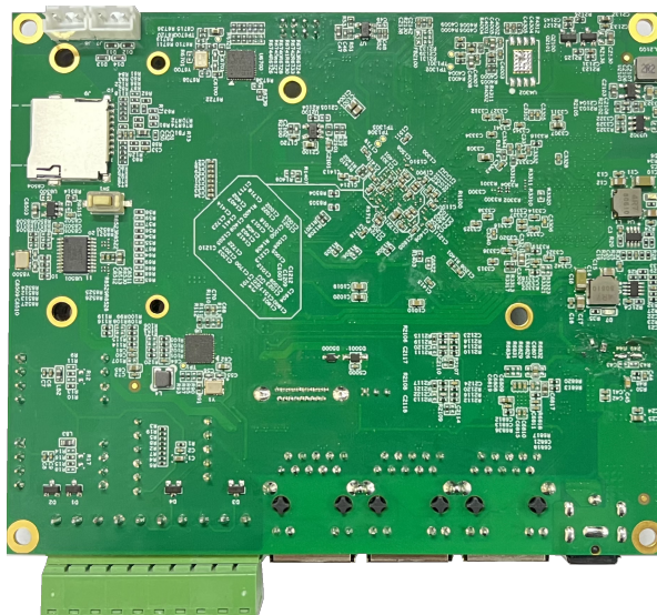
RK3568 定制开发板-背面图
